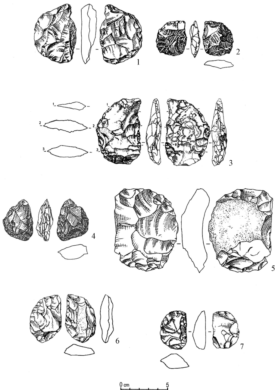
Рис. 3. Изделия D-образной формы: Черкасское (1–2, 4), Марьева Гора (3, 5), Семибалки (6–7). По: Колесник, Весельский 2005; Данильченко и др. 2020; Колесник и др. 2022
