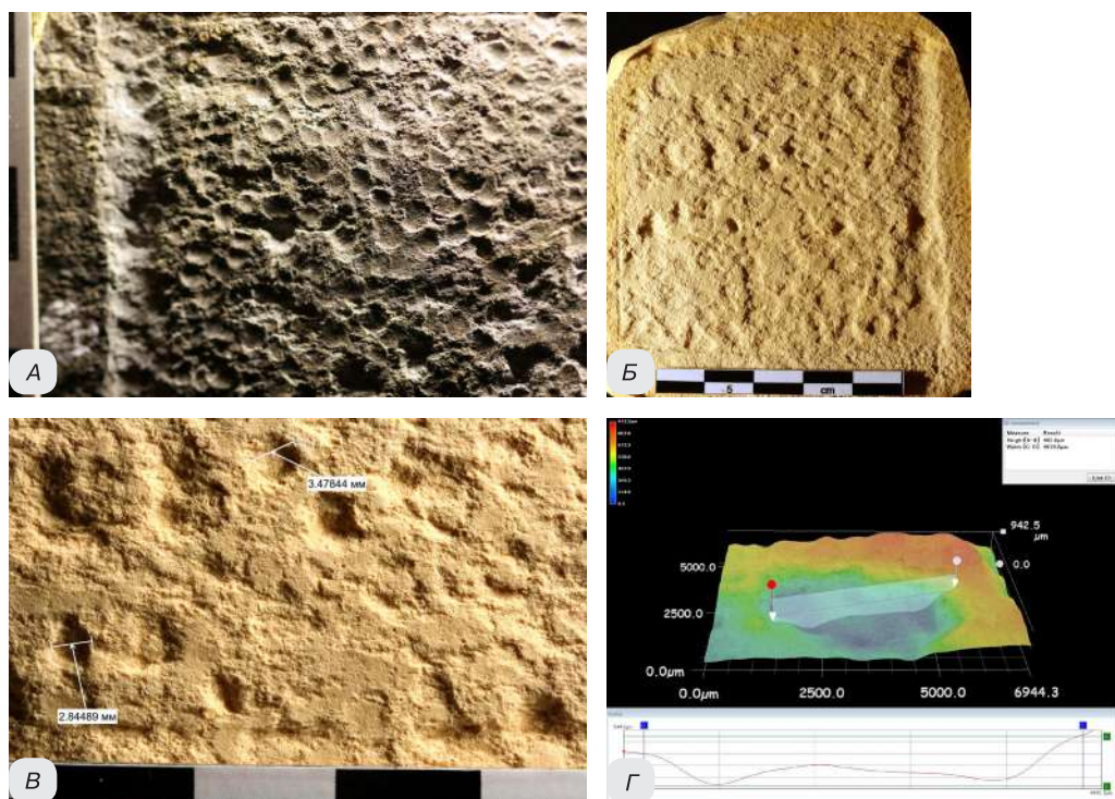
Рис. 19. Следы экспериментальной обработки пикетажем поверхности среднезернистого песчаника с начальной стадией развития корки выветривания, выполненной бронзовым заостренным стержнем, использованным в качестве посредника: А — вид следов на поверхности породы, косонаправленное круговое освещение, полученное в поле с помощью гибкой кольцевой бленды; Б — гипсовая отливка, полученная в поле с помощью гибкой кольцевой бленды; В — вид следов обработки на поверхности гипсовой отливки; Г — профиль следов обработки
