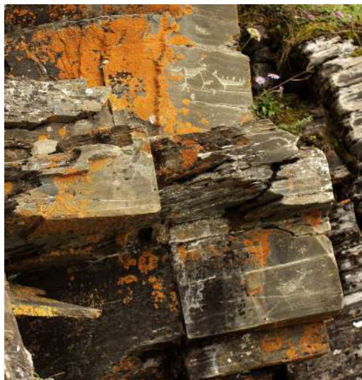
Рис. 3. Следы разрушения скального массива Кайкуульского обрыва на ортогональные блоки в результате избыточного, превышающего предел прочности породы, изгиба Fig. 3. Traces of destruction of the Kaikuul cliff massif into orthogonal blocks as a result of excessive bending exceeding the rock strength limit
