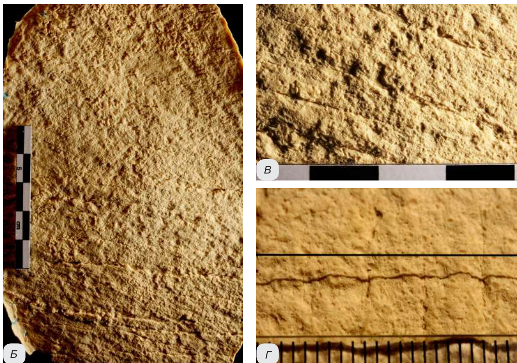
Рис. 23 (окончание). Б — гипсовая отливка, полученная с силиконового слепка обработанной поверхности, демонстрирующая слабо изменённую неглубоким разреженным пикетажем естественную исходную поверхность; В — вид следов обработки (неглубокого разнофигурного разреженного пикетажа) на поверхности гипсовой отливки; Г — профиль следов обработки (пикетажа)
