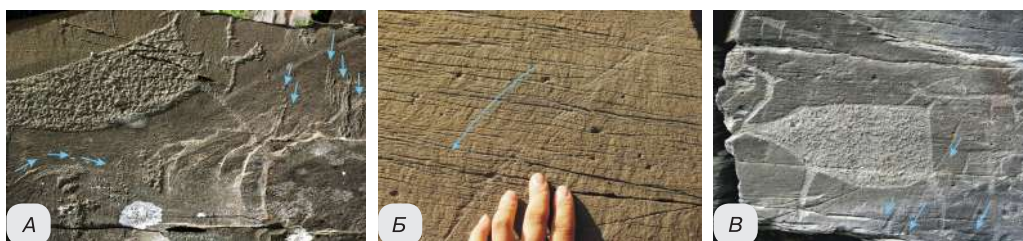
Рис. 13. А — разнонаправленные сбросовые штрихи, царапины и линейная шлифовка, наблюдаемые на поверхности крупного песчаного блока, происходящие от столкновения блоков в ходе камнепада. Стрелками указаны направления воздействий; Б — сбросовые штрихи, царапины и линейная шлифовка, наблюдаемые на песчаной поверхности сброса-скольжения на скале склона Кайкуульского обрыва, имитирующие следы обработки; В — изображение оленей, выполненное пикетажем поверх следов сброса-скольжения
