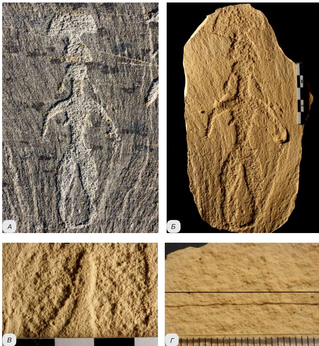
Рис. 33. А — изображение «женщины-мухомора», интерпретируемое нами как выполненное пикетажем на поверхности среднезернистого песчаника в начальной стадии развития корки выветривания с помощью посредника из закалённого железа, прямое фронтальное освещение. Б — гипсовая отливка, полученная с силиконового слепка обработанной поверхности. В — вид следов обработки на поверхности гипсовой отливки; Г — профиль следов обработки
